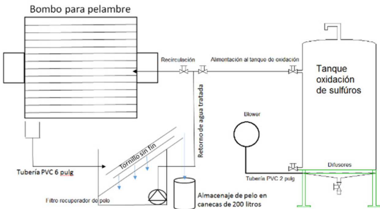
Figura 2. Esquema del sistema de oxidación de sulfuros.
